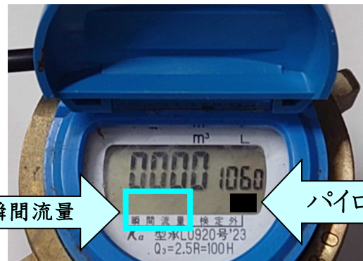
電子式水道メーター
